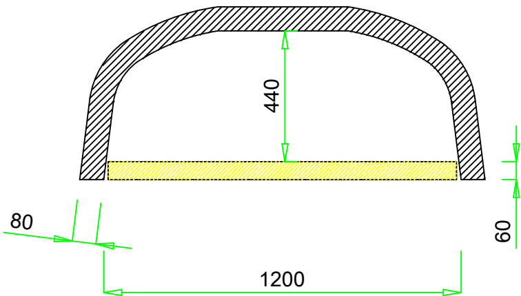
Sezione A-A
